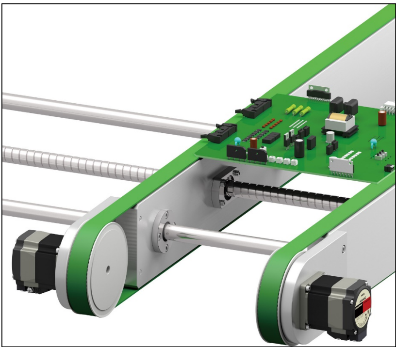
สายพานลำเลียงคู่ที่ต้องทำงานพร้อมกัน
